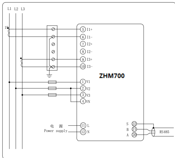
图 7.4.3 三相三线系统：2LL、2CT 接线
